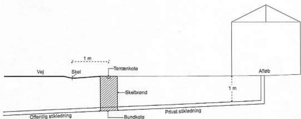
Situationskitse for tilslutning til offentlig kloak.
